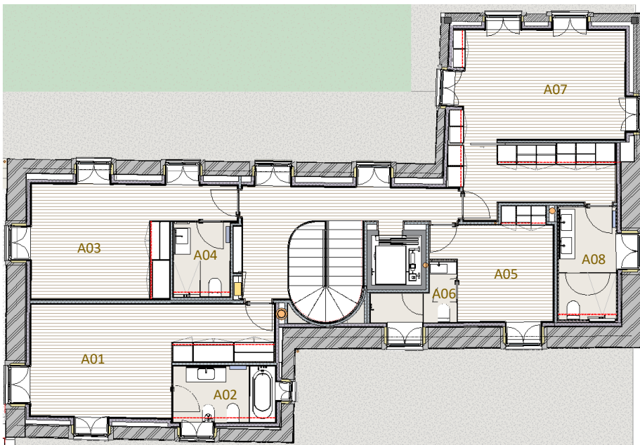
PISO 2 | VOLUME B
